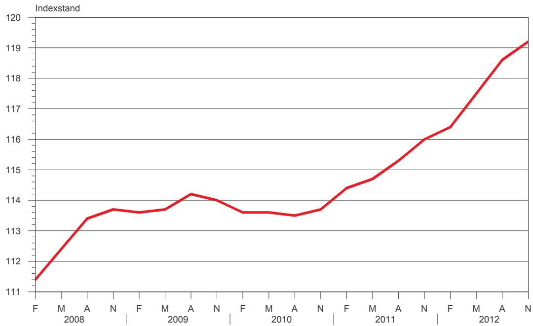
Entwicklung des Preisindex für den Straßenbau 2005 = 100
