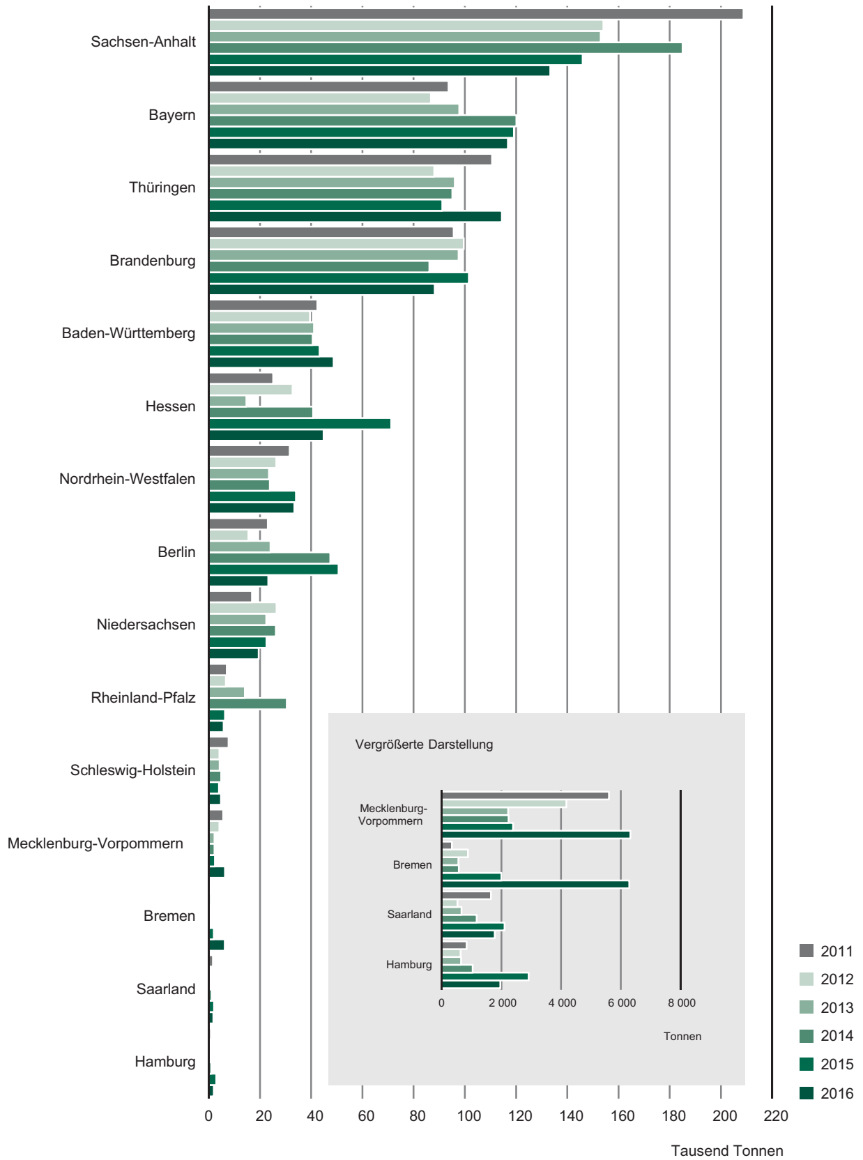
Abb. 8 Aus anderen Bundesländern angenommene und in Sachsen entsorgte gefährliche Abfallmengen 2011 bis 2016
