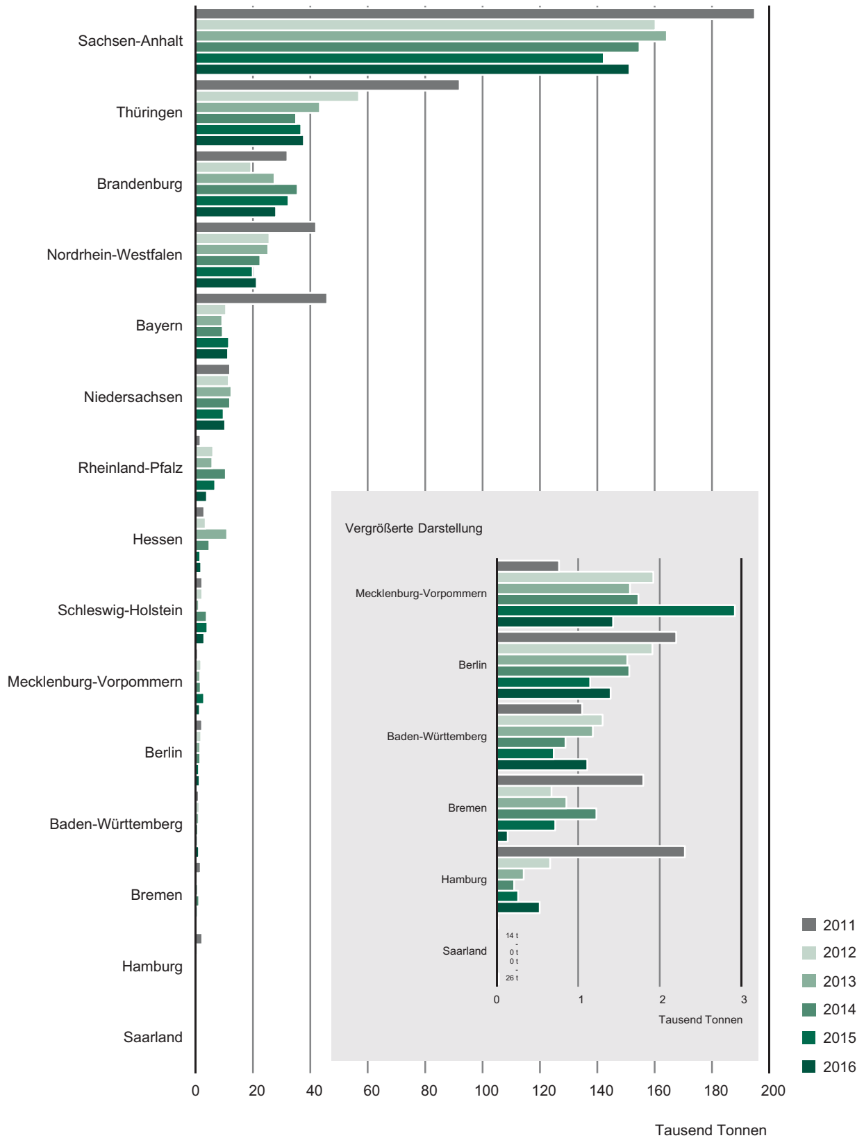
Abb. 7 In Sachsen erzeugte und in andere Bundesländer abgegebene gefährliche Abfallmengen 2011 bis 2016
