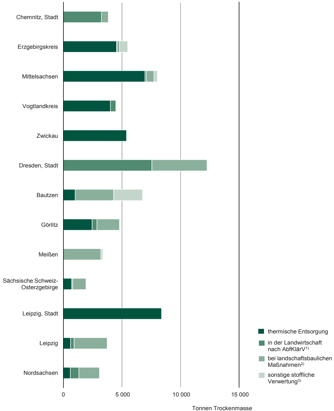
Abb. 3 Direkte Klärschlamm entsorgung aus öffentlichen biologischen Abwasserbehandlungsanlagen in Sachsen 2016 nach Entsorgungswegen und nach Kreisfreien Städten und Landkreisen
