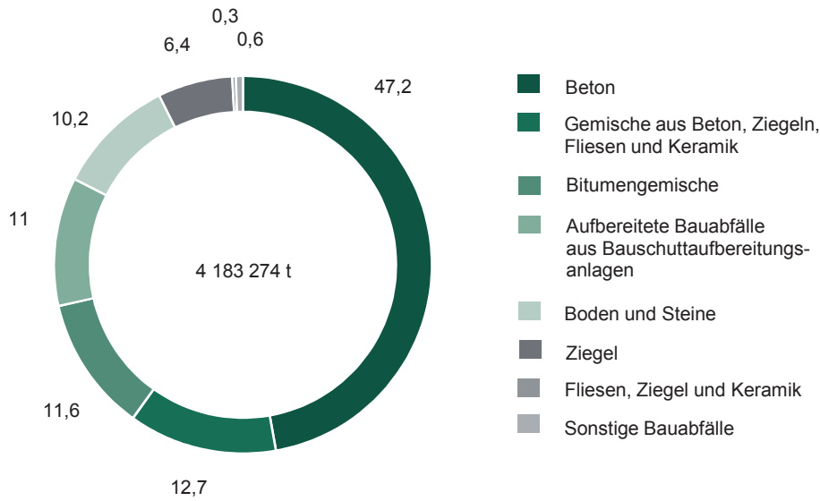
Abb. 3 In Aufbereitungsanlagen für Bauabfälle eingesetzte Bauabfälle 2012 in Prozent
