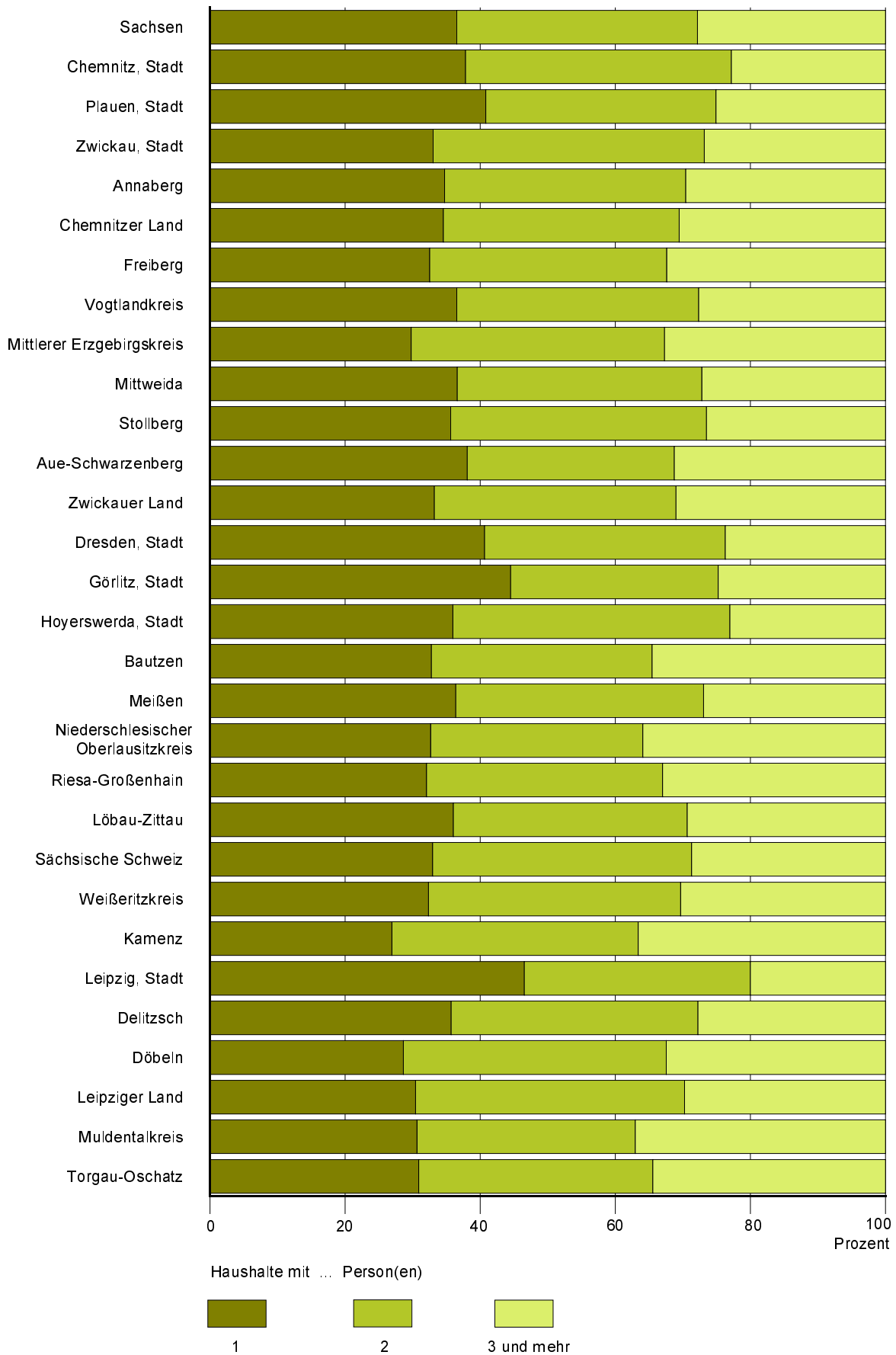
Abb. 5 Haushalte im April 2002 nach Haushaltsgröße und Kreisen
