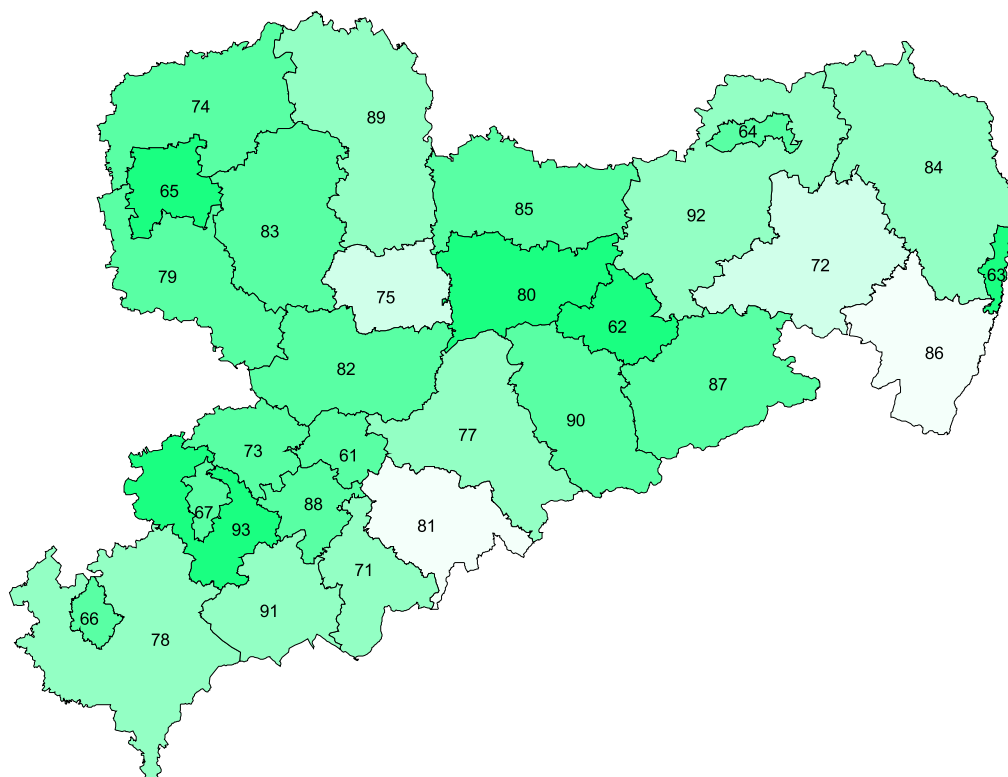
Abb. 4 Erwerbstätige im April 2002 nach durchschnittlichem Nettoeinkommen und Kreisen
