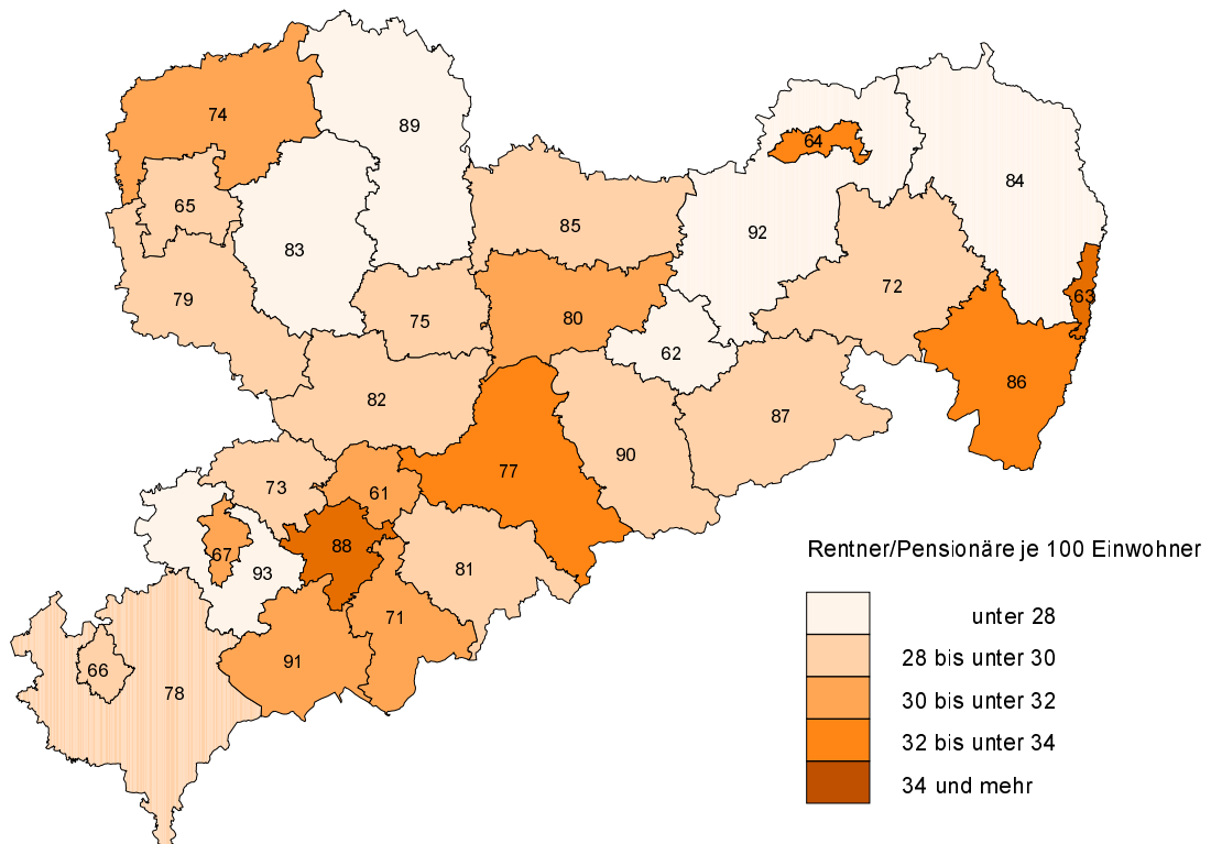
Abb. 2 Bevölkerung mit überwiegender Lebensunterhalt durch Rente/Pension je 100 Einwohner im April 2002 nach Kreisen
