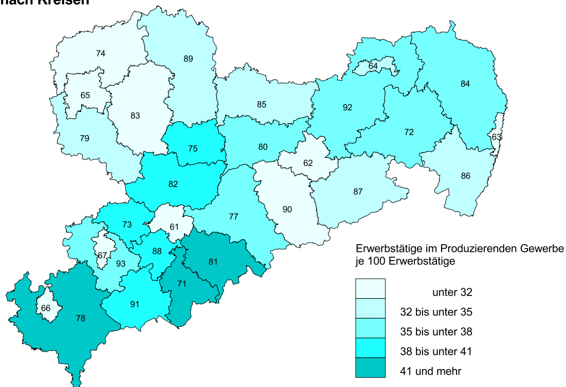
Abb. 3 Erwerbstätige im Produzierenden Gewerbe je 100 Erwerbstätige im April 2002 nach Kreisen
