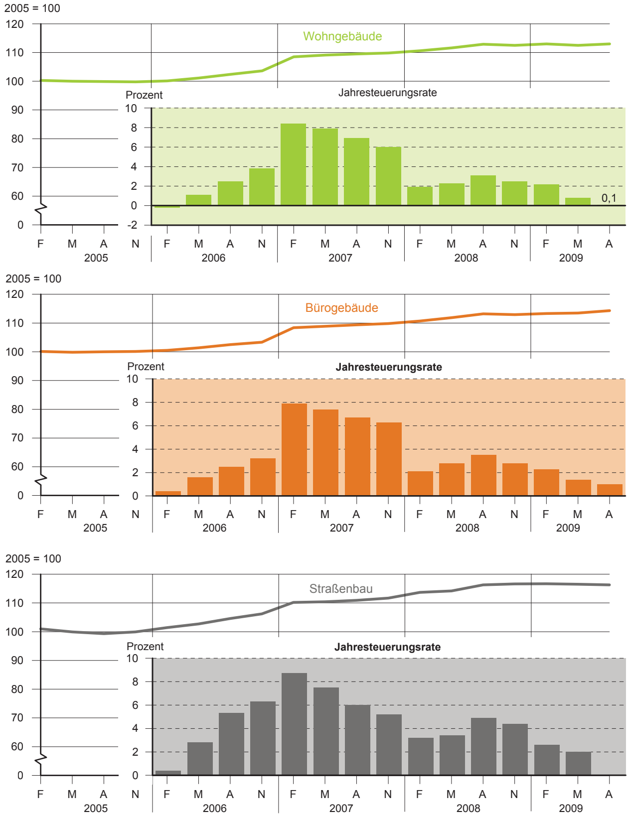
Abb. 1 Preisindizes für Bauwerke 2005 bis 2009
