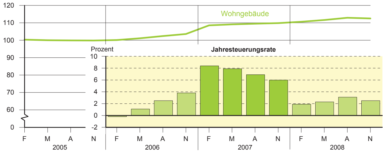
Abb. 1 Preisindizes für Bauwerke 2005 bis 2008
