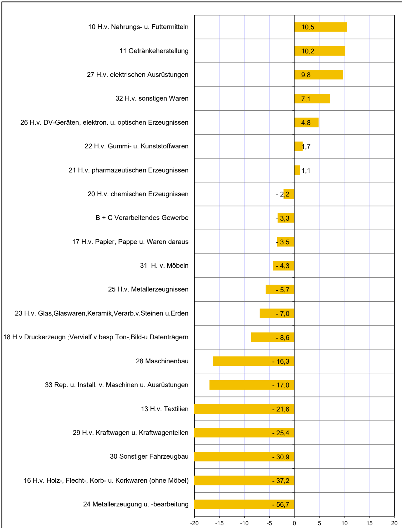
Grafik 3: Umsatz der Betriebe im Verarbeitenden Gewerbe sowie Bergbau und Gewinnung von Steinen und Erden in Schleswig-Holstein im Dezember 2019 Veränderung in ausgewählten Wirtschaftszweigen gegenüber dem Vorjahresmonat in % (Vorläufige Ergebnisse)
