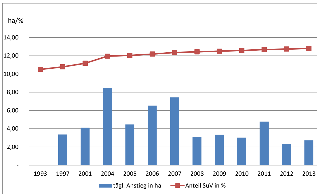
Grafik 2: Veränderung der Siedlungs- und Verkehrsfläche in Schleswig-Holstein von 1993 bis 2013
