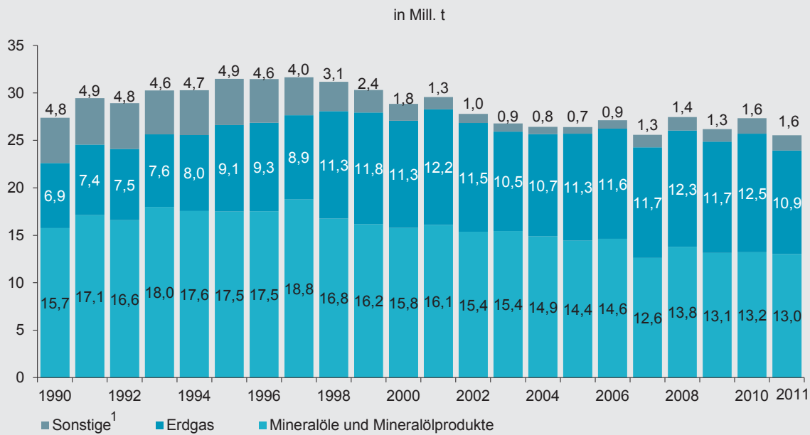
G 12 CO 2 -Emissionen aus dem Primärenergieverbrauch (Quellenbilanz) 1990–2011 nach Energieträgern
