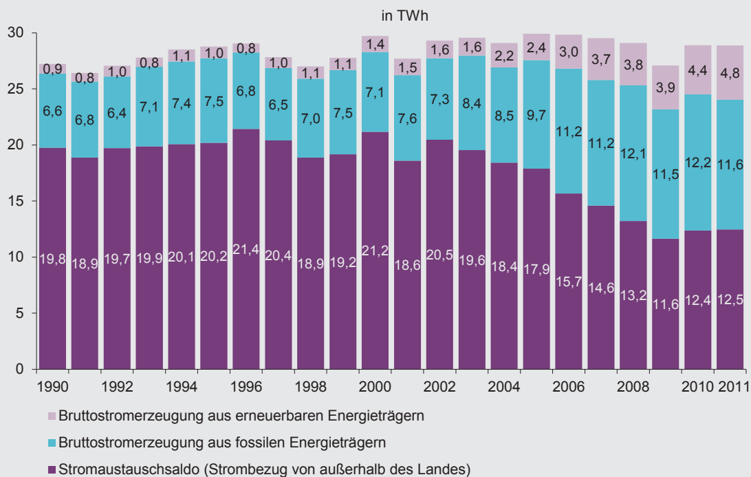
G 8 Struktur des Bruttostromverbrauchs 1990–2011
