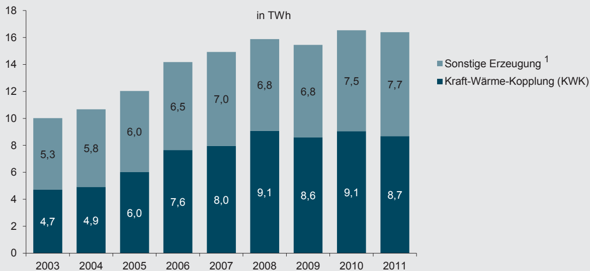
G 9 Bruttostromerzeugung 2003–2011 nach Art des Gewinnungsprozesses
