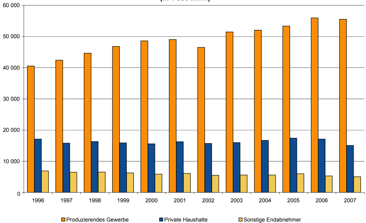
Gasabsatz nach Verbrauchergruppen 1996 bis 2007 (in 1 000 MWh)
