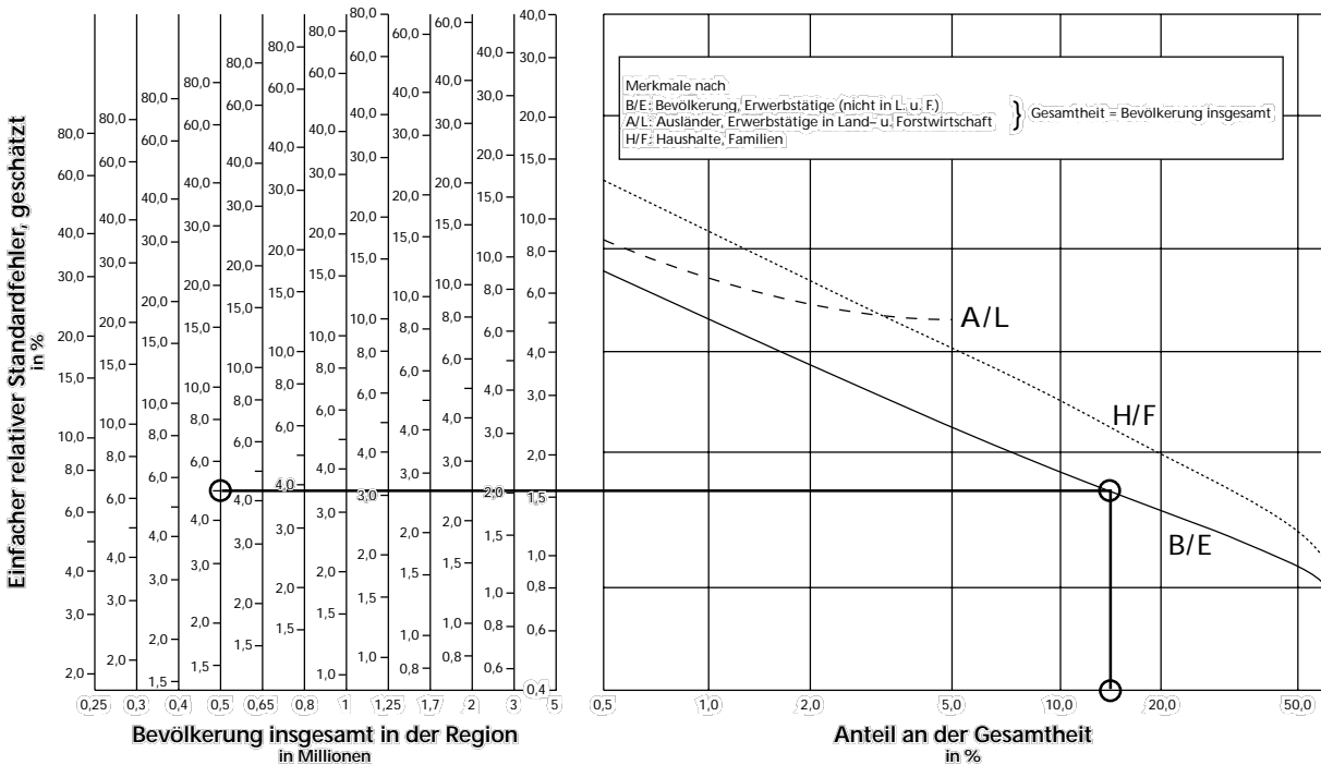
Einfacher Standardfehler der 1% – Mikrozensusstichprobe 1) für unterschiedliche Regionsgrößen
