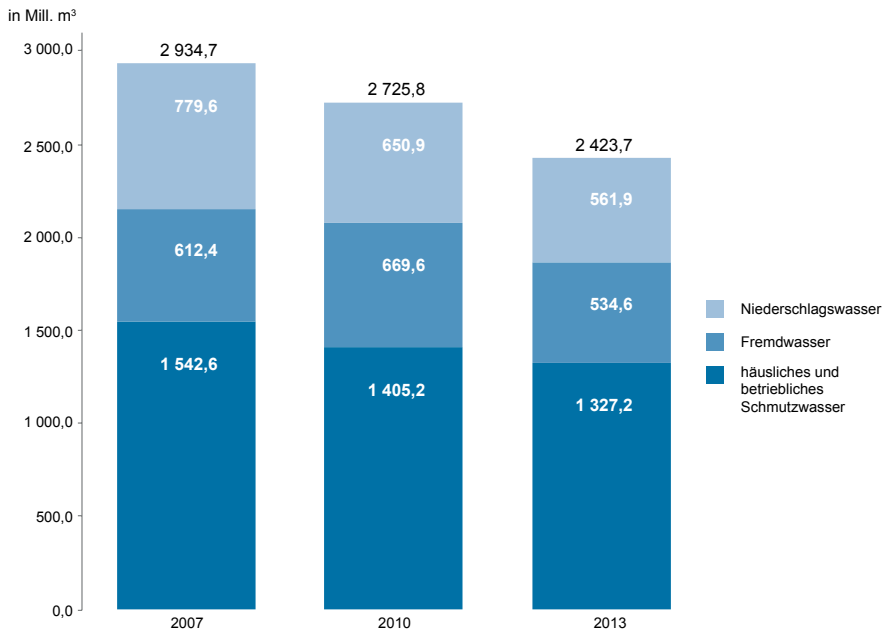
Abb. 1 Abwassermengen in NRW 2007, 2010 und 2013 nach Abwasserart
