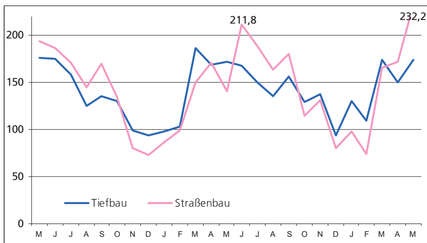
Tiefbau
