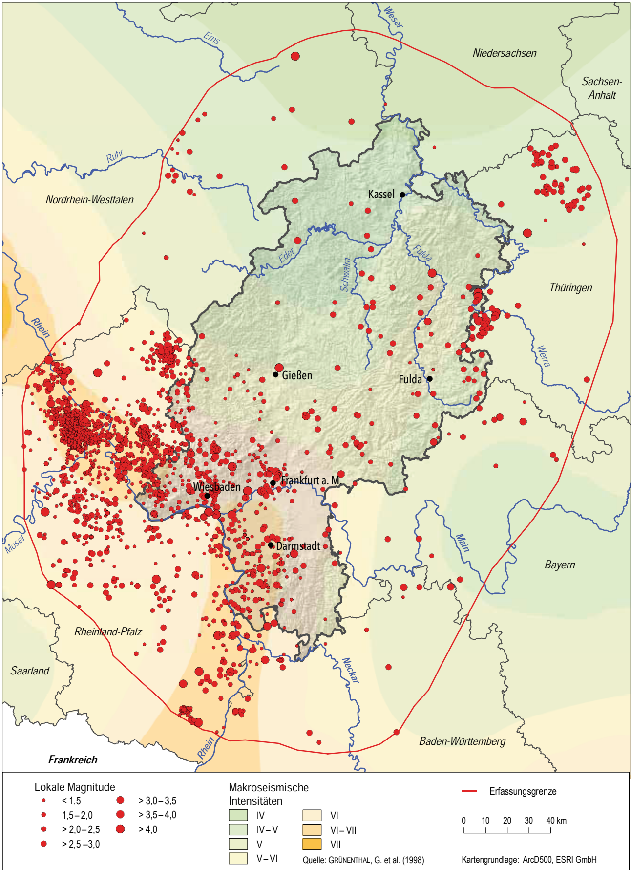
Abb. 2: GIS-Darstellung des seismischen Kataloges Hessen (SKHe2012) für den Zeitraum 858–Dezember 2011.
