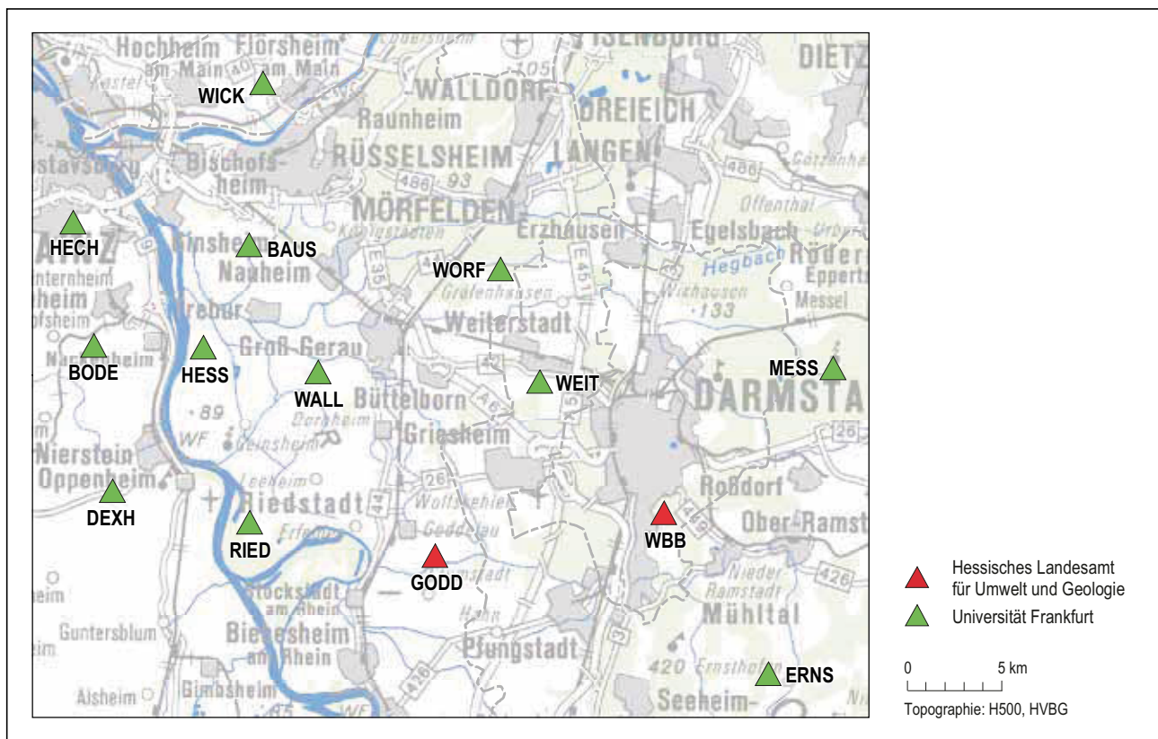
Abb. 2: Netz der Messtationen im Untersuchungsgebiet zur Registrierung der natürlichen Seismizität im Verbundprojekt SiMoN.
