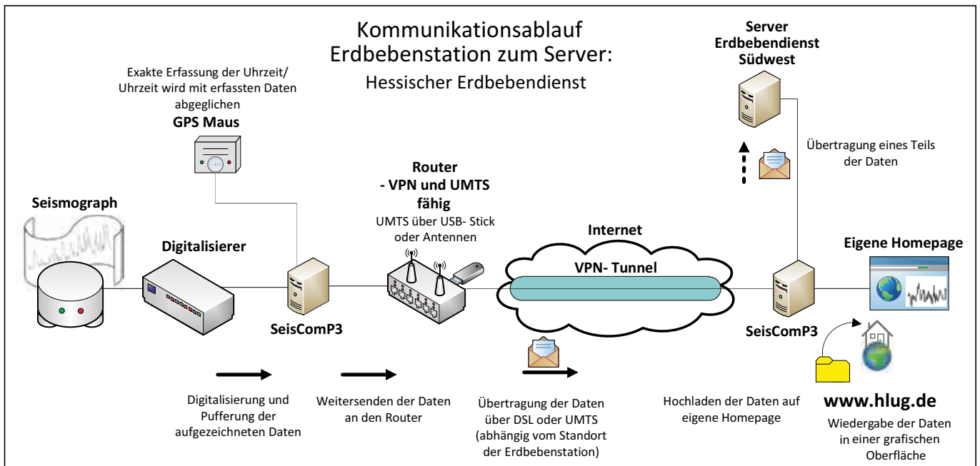
Abb. 4: Kommunikationsablauf der im Verbundprojekt SiMoN gewonnenen Daten.
