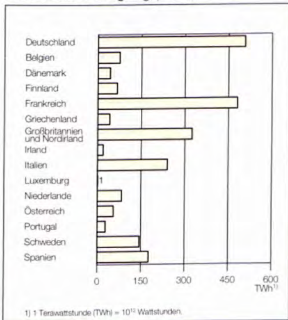
Elektrizitätserzeugung (netto) 1997
