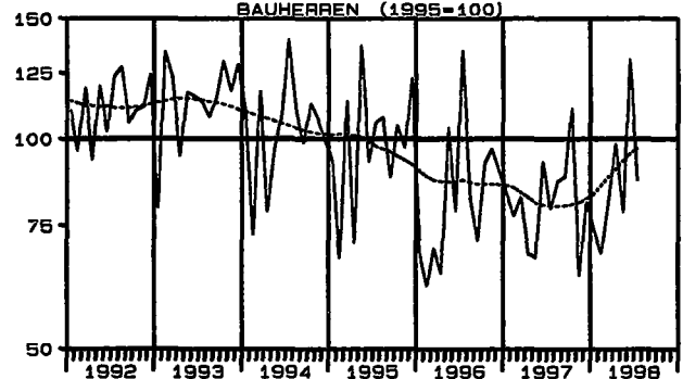
RAUMINHALT IM NICHTWOHNBAU - NICHTOEFFENTLICHE BAUHERREN (1995=100)
