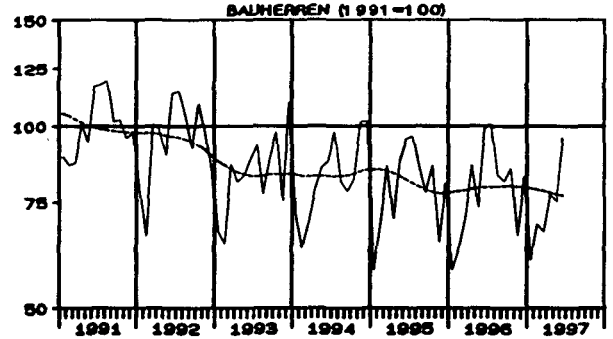
RAUMINHALT IM NICHTWOHNBAU - NICHTOEFFENTLICHE BAUHERRN (1991=100)
