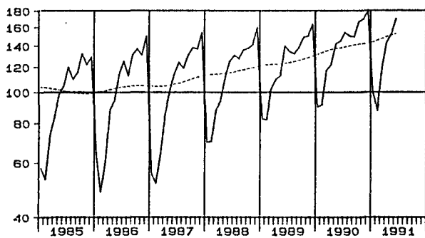
BAUGEWERBLICHER UMSATZ
