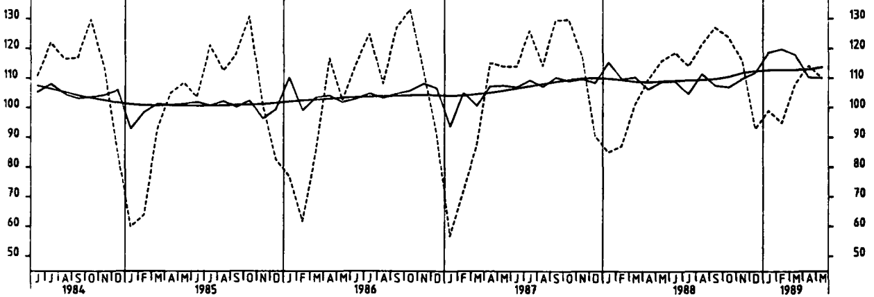
GELEISTETE ARBEITSSTUNDEN, GEWERBLICHER UND INDUSTRIELLER BAU, 1985=100
