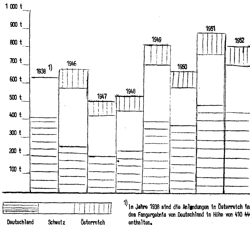
Anteile der Uferstaaten an den Gesamtfangmengen im Bodensee.
