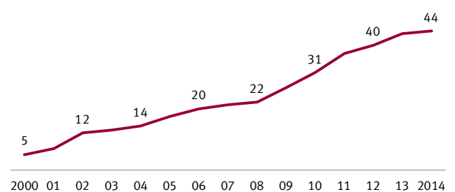
Internetnutzer je 100 Einwohner
