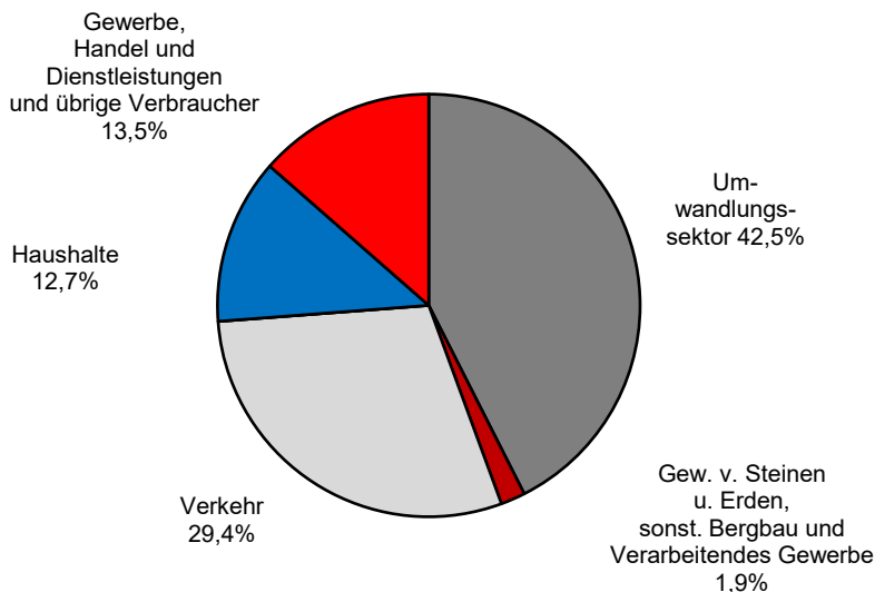
Anteil der CO 2 -Emissionen (Quellenbilanz) nach Sektoren 2023
